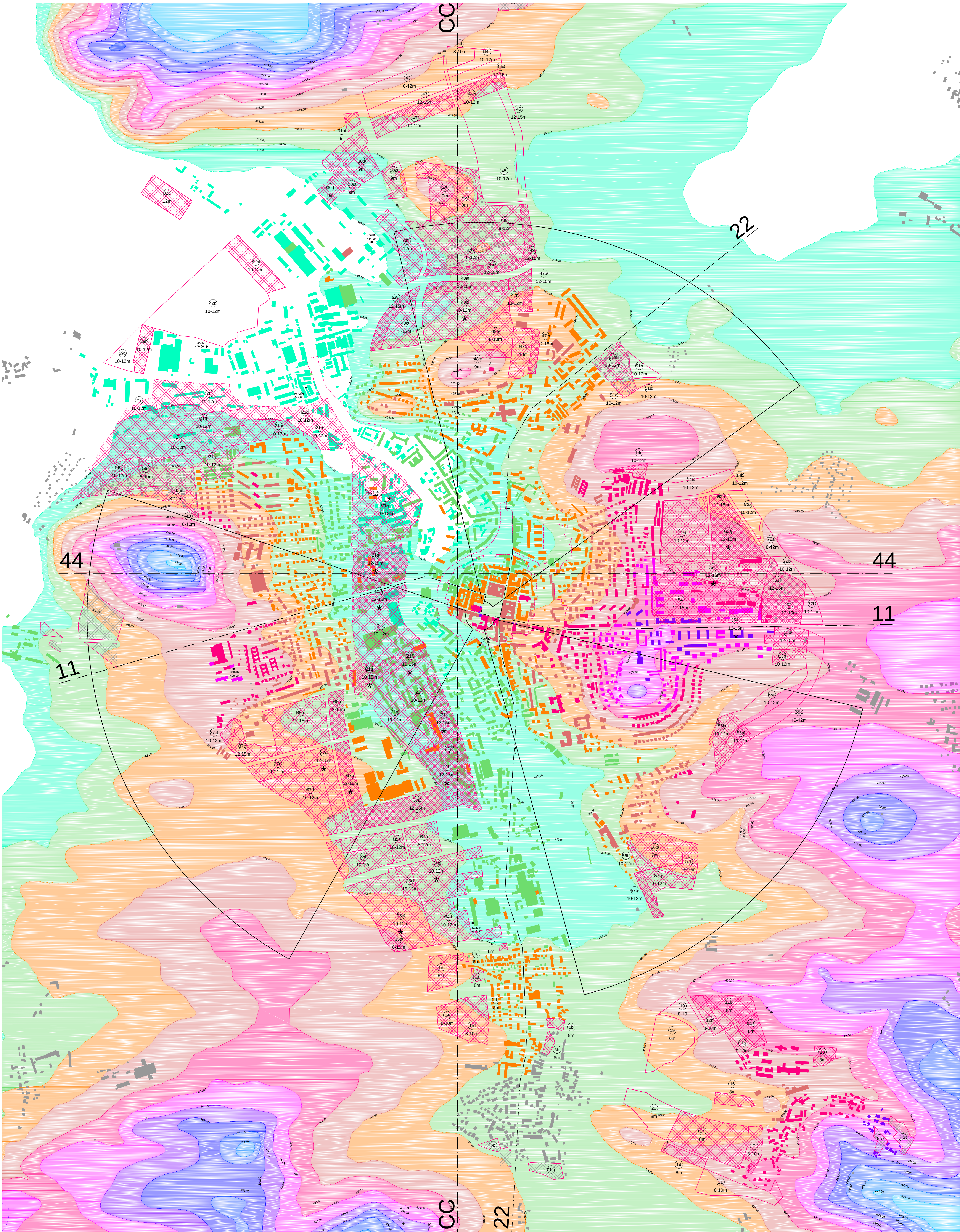
SITUACE SCHÉMATU VÝŠKOVÉ REGULACE M 1:8000
