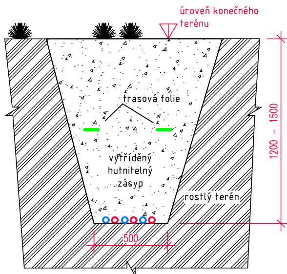
ŘEZ A-A
